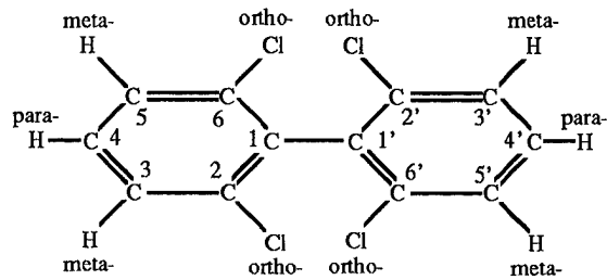
2,6,2',6' Tetrachlorobiphenyl
