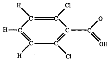
2,6 Dichlorobenzoic acid
